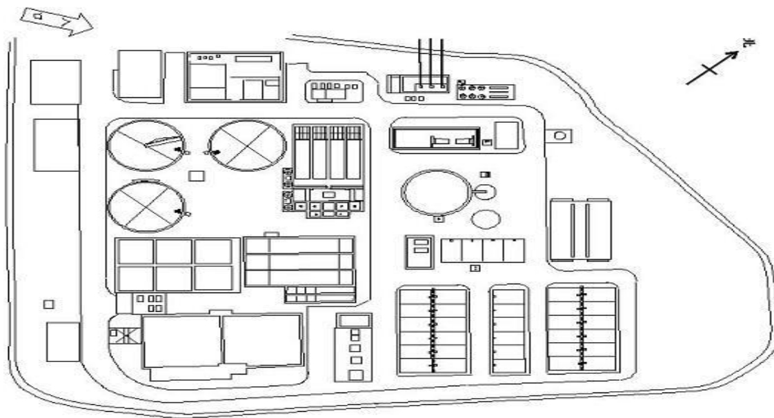
工業區污水處理廠平面配置圖
