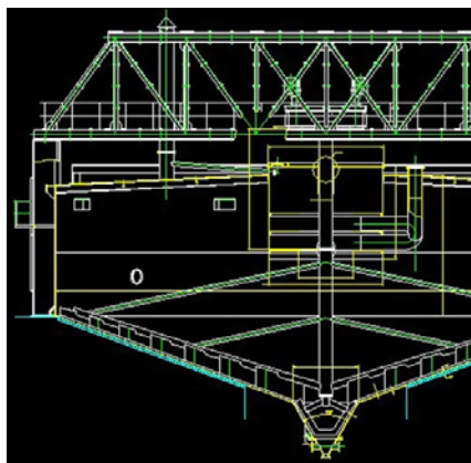
沉降槽機械視圖
